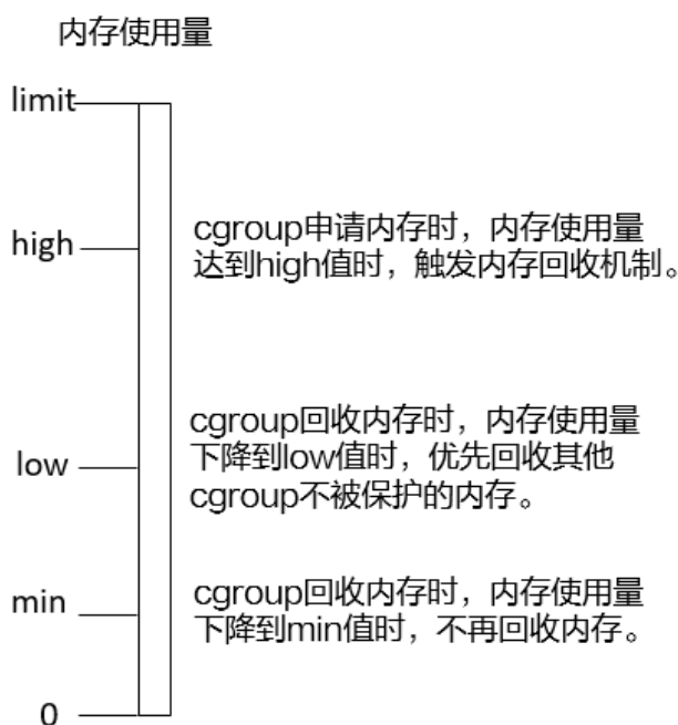
图 10-5 内存回收机制
