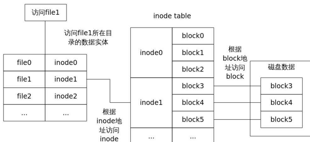
图 10-2 EXT4 文件系统结构
